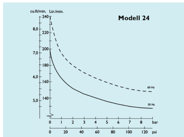
Jun-Air Kompressor 24-40
