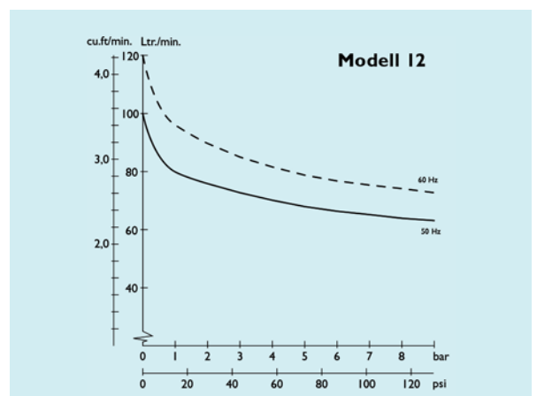
Jun-Air Kompressor 12-40
