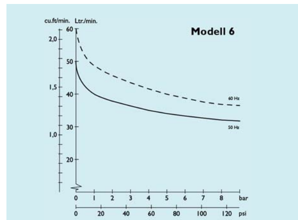
Jun-Air Kompressor 6-15
