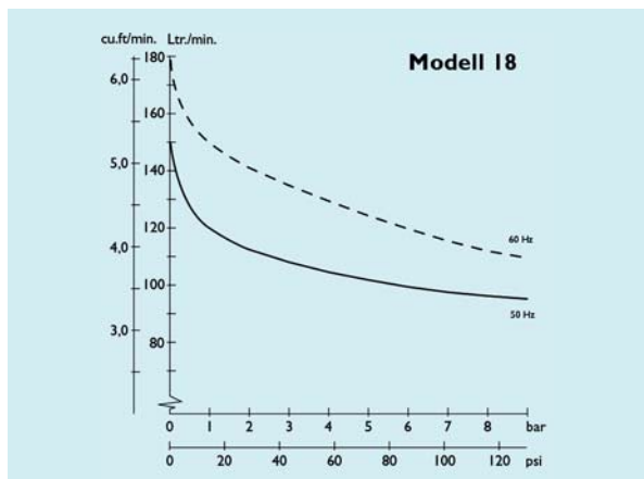
Jun-Air Kompressor 18-40
